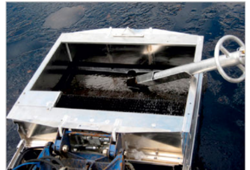
Der Doro Skimmer kann sowohl mit als auch ohne Sala Walzpumpe verwendet werden. Der Doro Skimmer fasst ungefähr 20 Liter.
